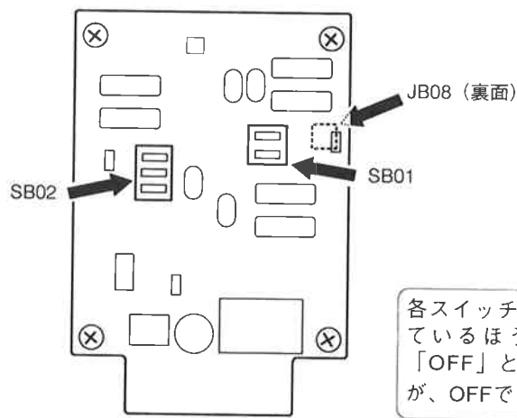
部品配置図
